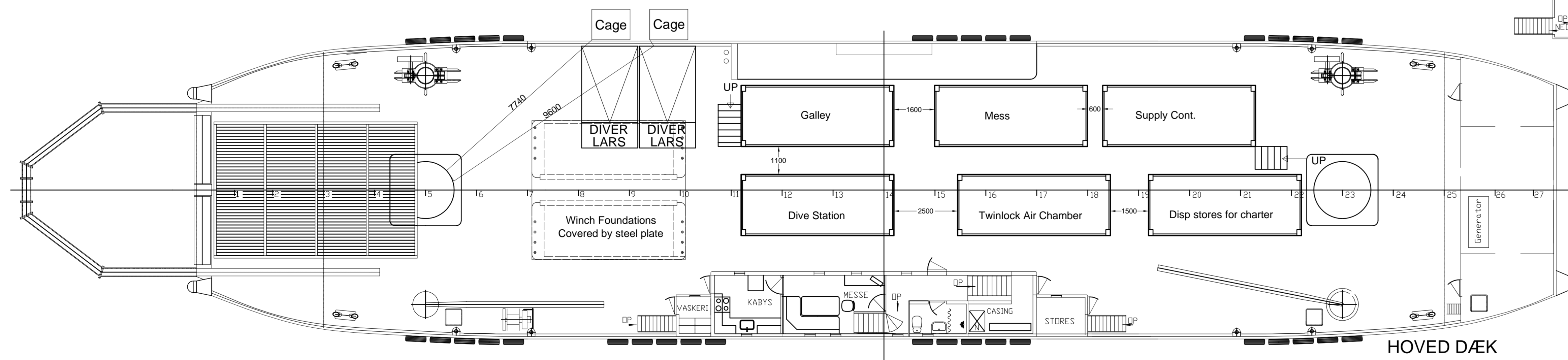
HOVED DÆK
