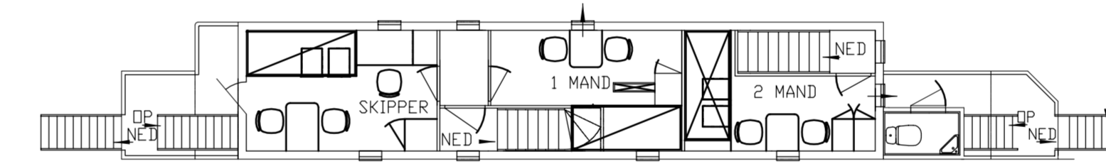
A - DÆK
